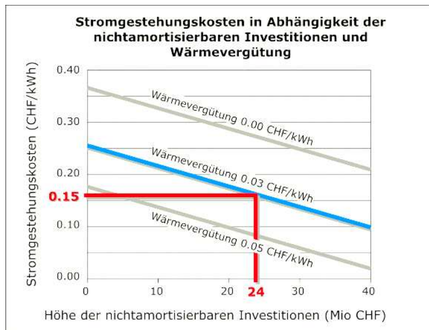
Fig. 13: Stromgestehungskosten
