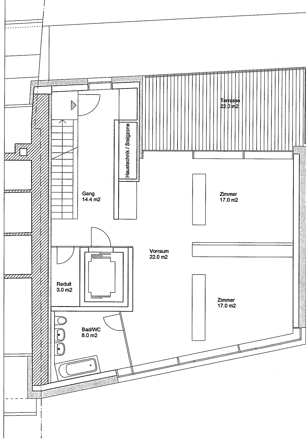
5. OG Wohnung
