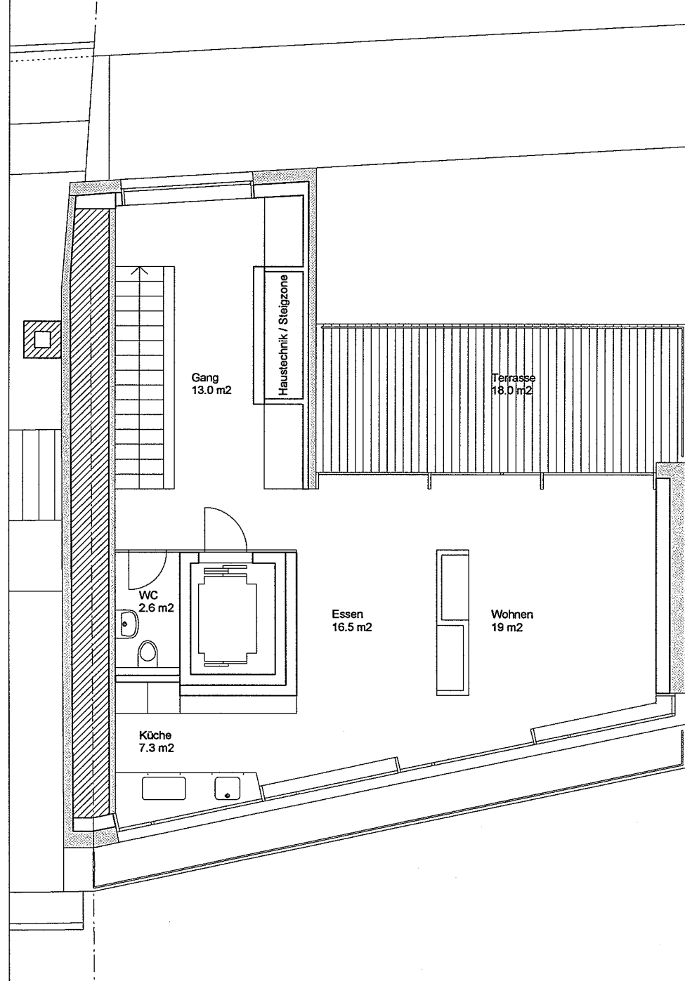
DG Wohnung
