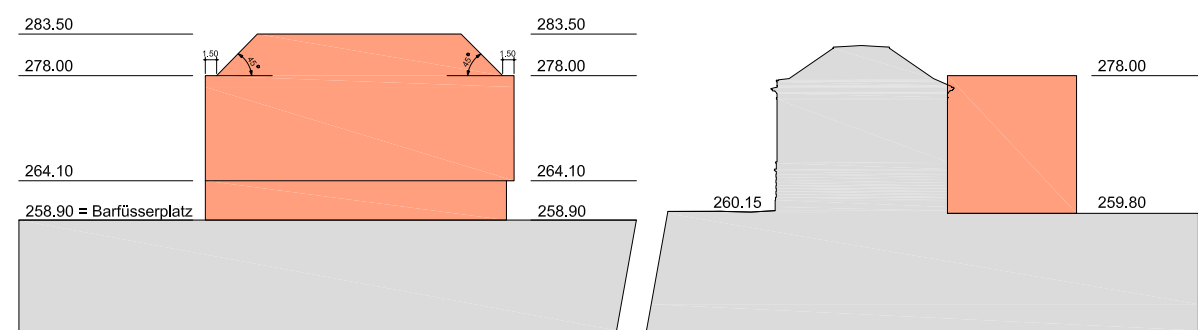
Profil West
