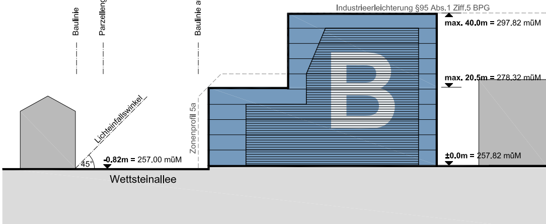
Typ B Schnitt A-A
