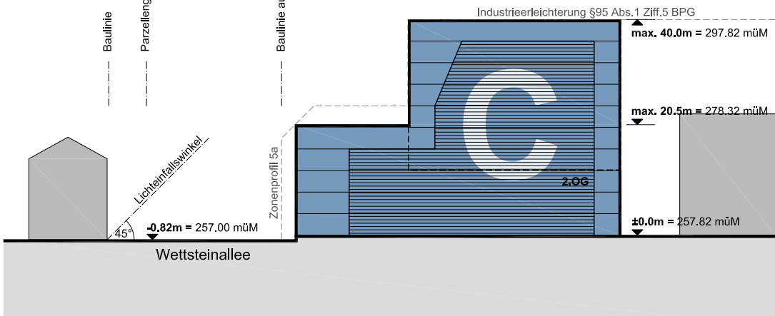
Typ C Schnitt A-A
