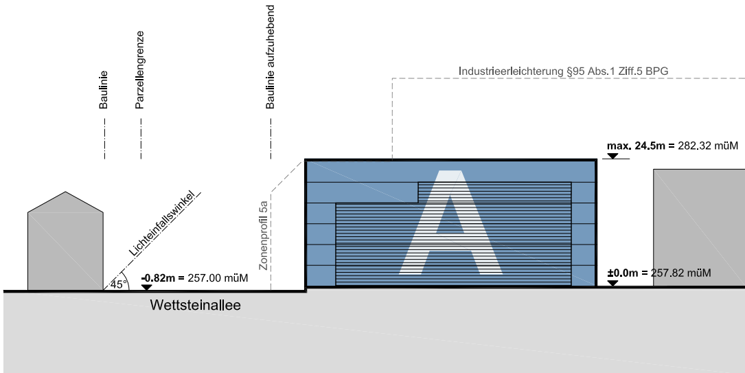
Typ A Schnitt A-A
