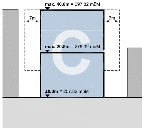
Typ C Ansicht Nord
