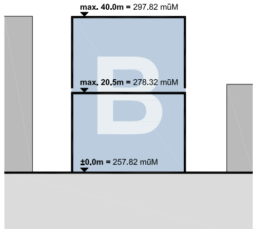
Typ B Ansicht Nord
