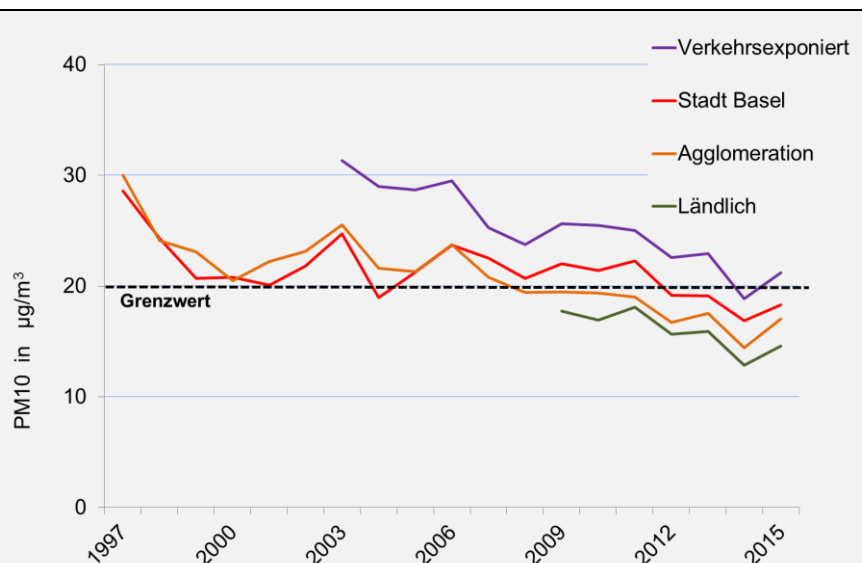
Abb. 12: Entwicklung der PM10-Jahresmittelwerte von 1997 bis 2015
