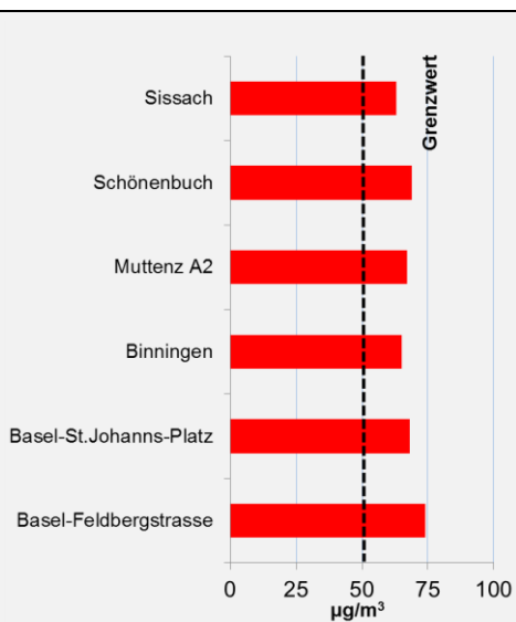
Abb. 11: Max. Tageswerte im 2015
