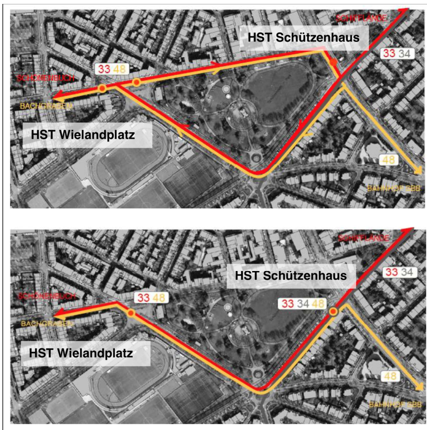
Abbildung 3: Führung Buslinien
