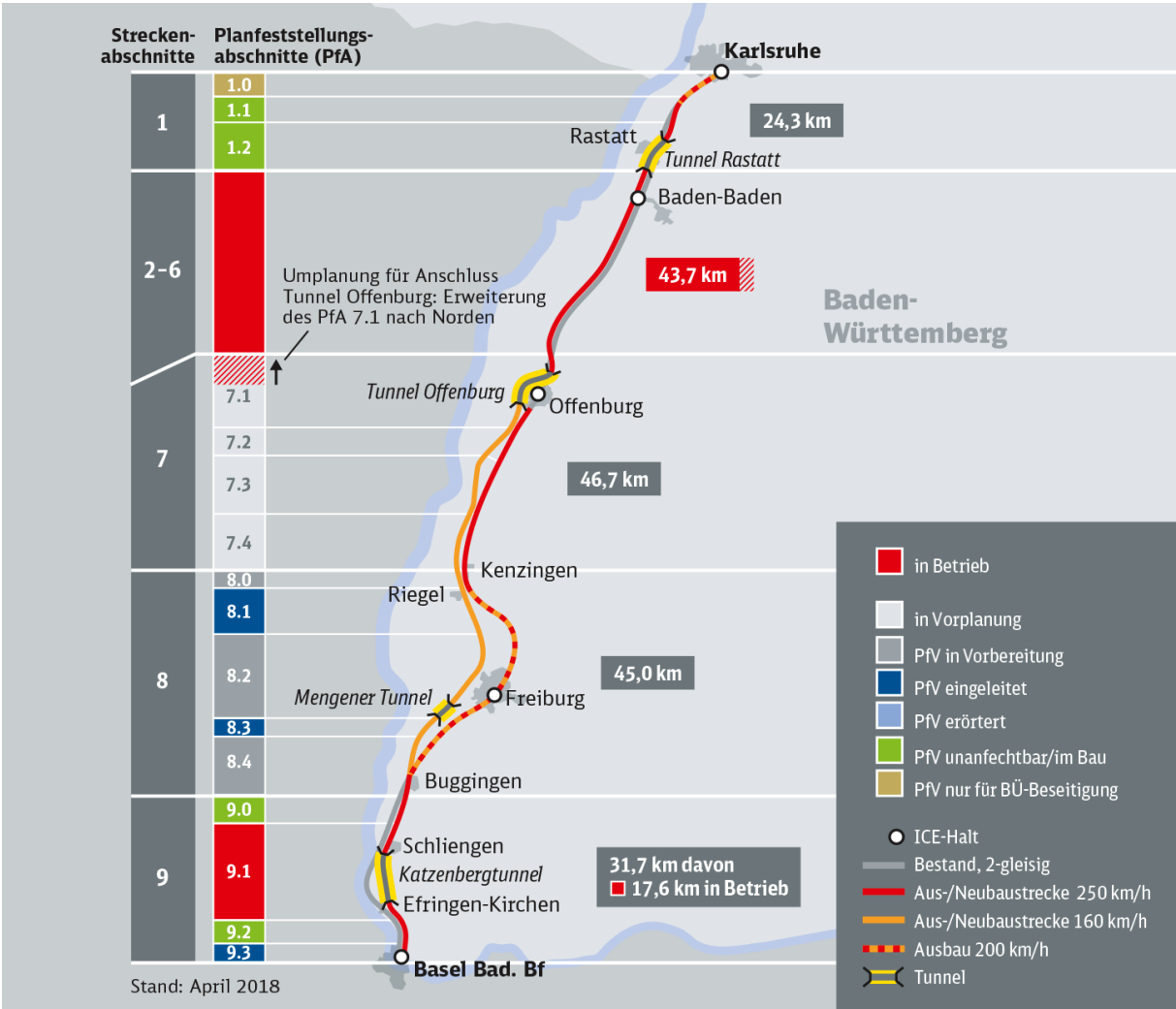
Abb. 19: Ausbau Oberrheinstrecke (Quelle: DB Netze AG, Stand April 2018)
